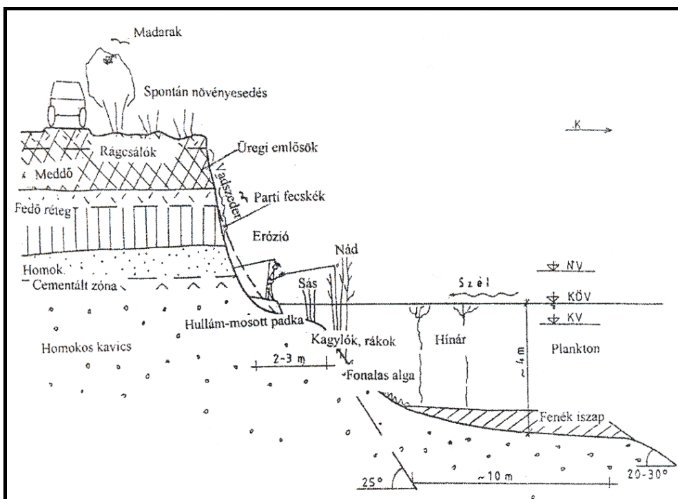
15. ábra: Horgászat számára megfelelő parti részsű szelvénye
