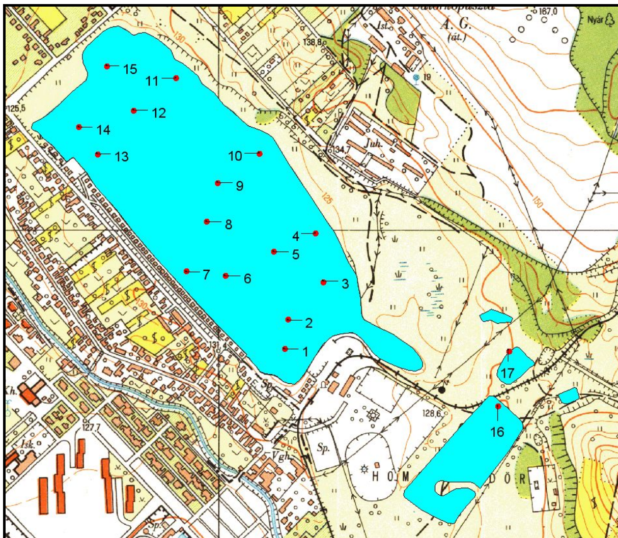
12. ábra: A Hydrolabos mérési pontok elhelyezkedése
