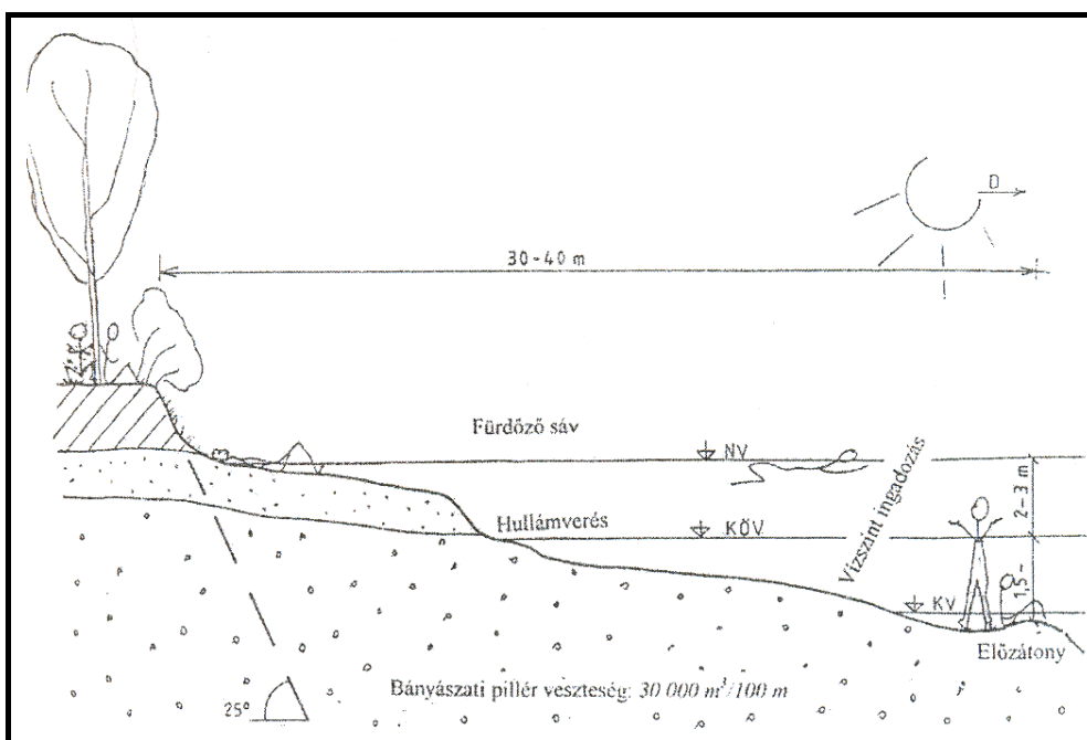
16. ábra: Fürdőzés számára kialakított parti részsű szelvénye
